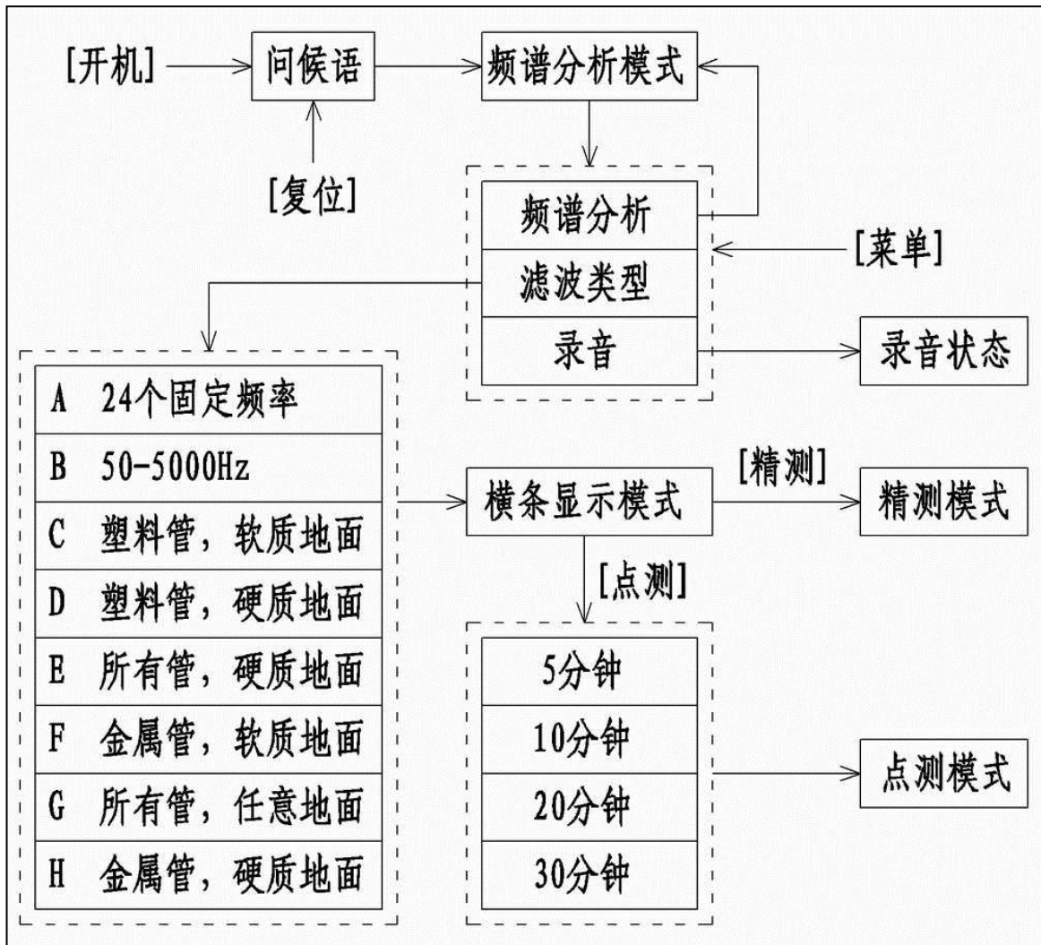
JT-5000 智能数字式漏水检测仪操作流程图中：
