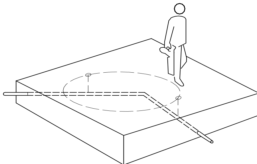
图 c 管道改变方向探测示意图
